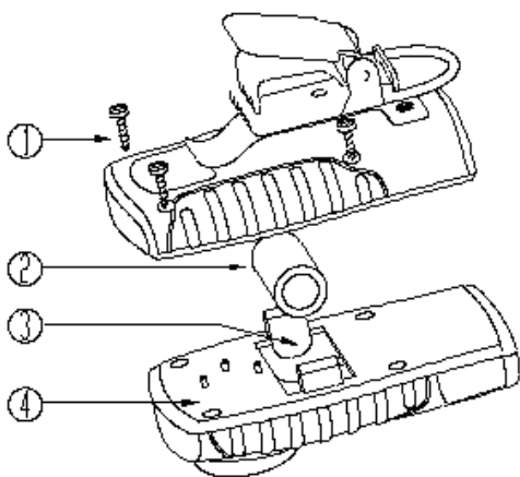
Замена батареи
