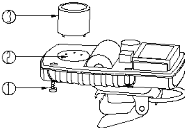
Замена датчика
