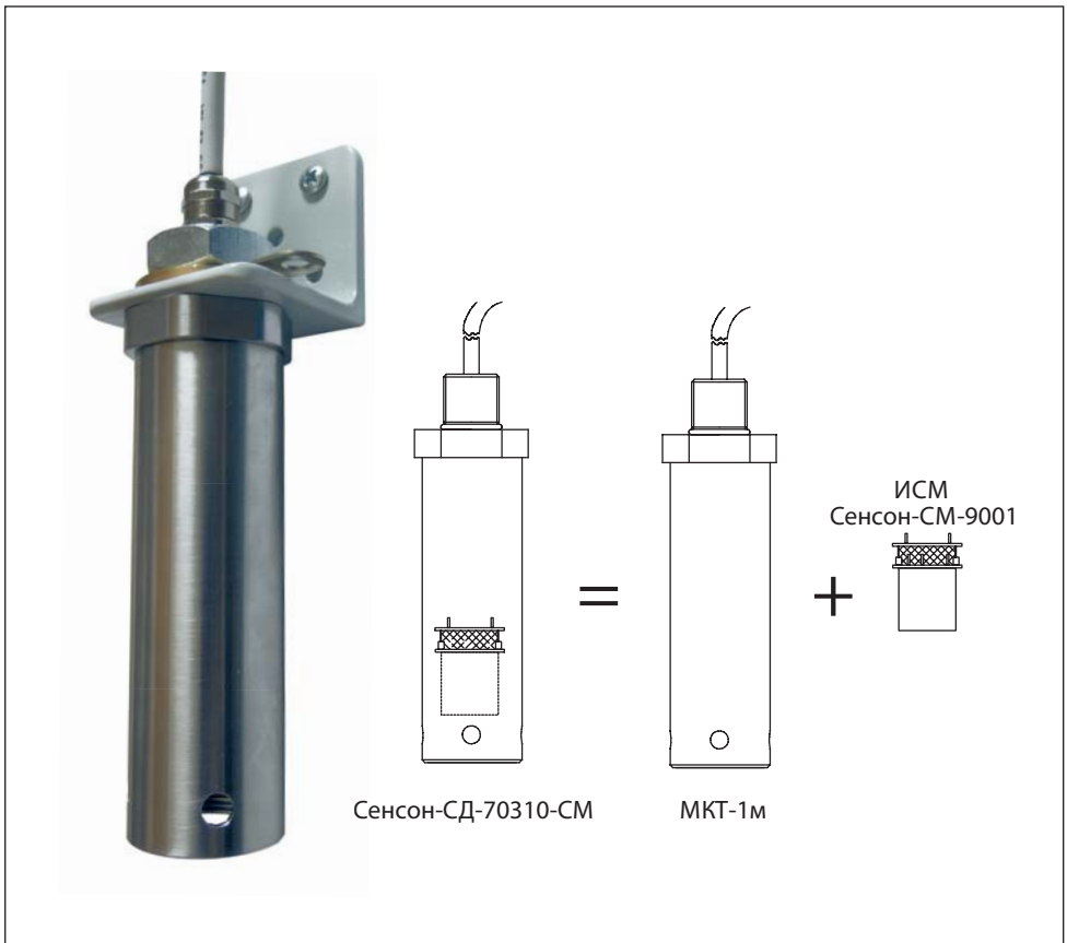
Рис.1. ГС "Сенсон-СД-7031-СМ"
