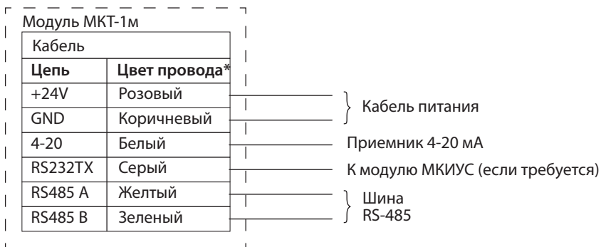
Рис.6. Схема подключения ГС "Сенсон-СД-7031-СМ"
