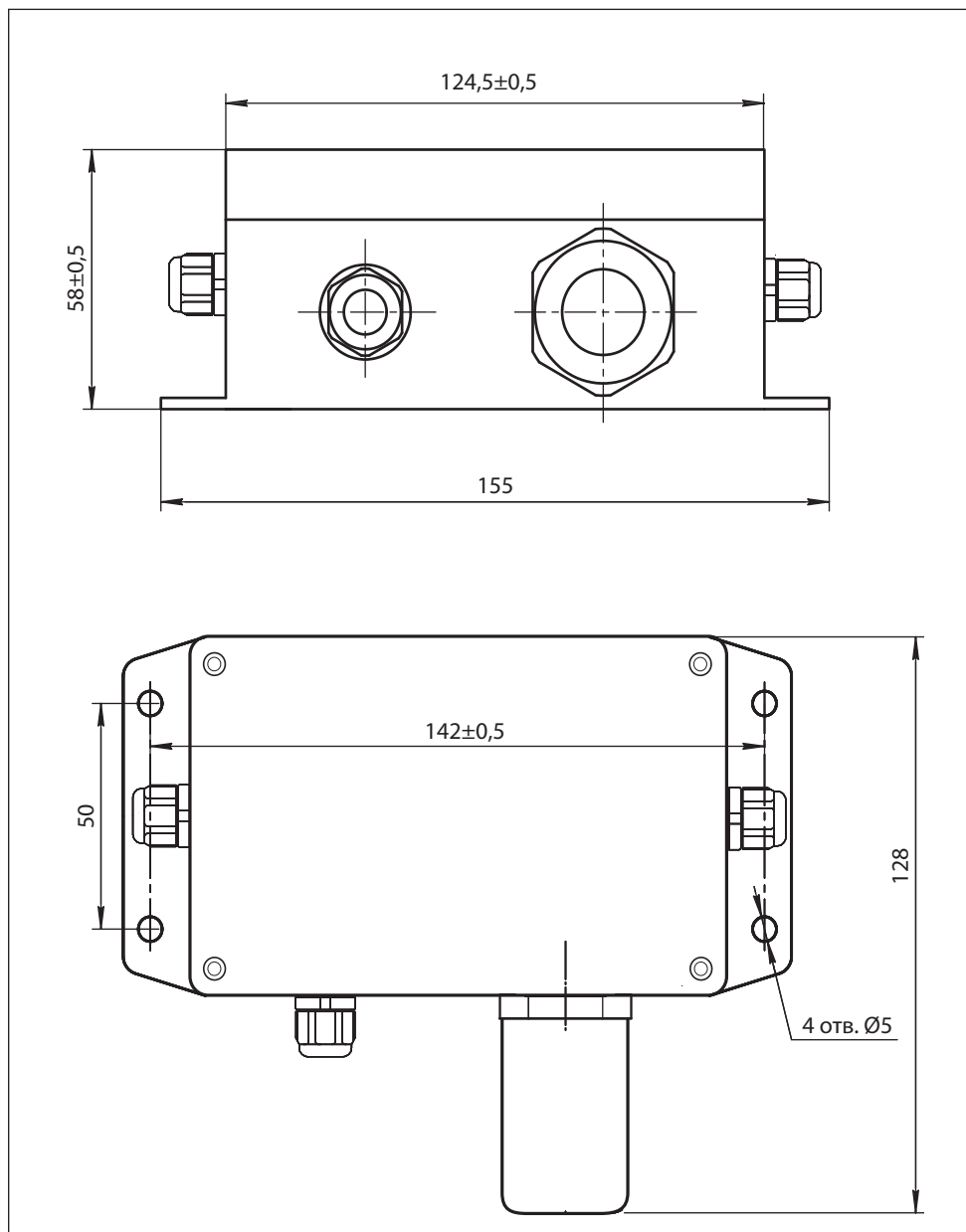
Рис.5. Габаритный чертеж ГС "Сенсон-СД-7033-СМ"
