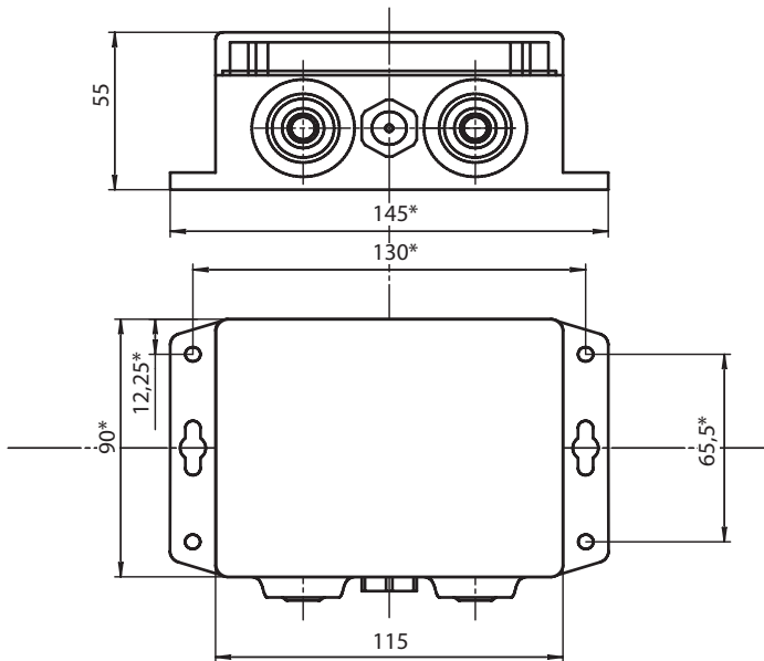
Рис.1. Габаритный чертеж контроллера "Сенсон К-1М"
