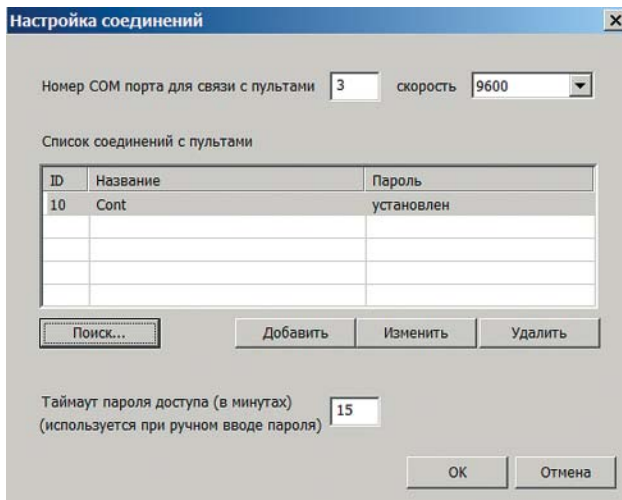
Рис. А2. Окно настройки соединений
