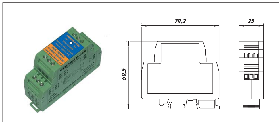
Рис.5. Сетевое реле "Сенсон Р-02Ц"
